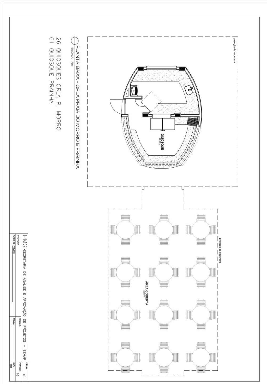
PLANTA BAIXA – QUIOSQUE PRAIA DOS NAMORADOS (ANEXO 2)
