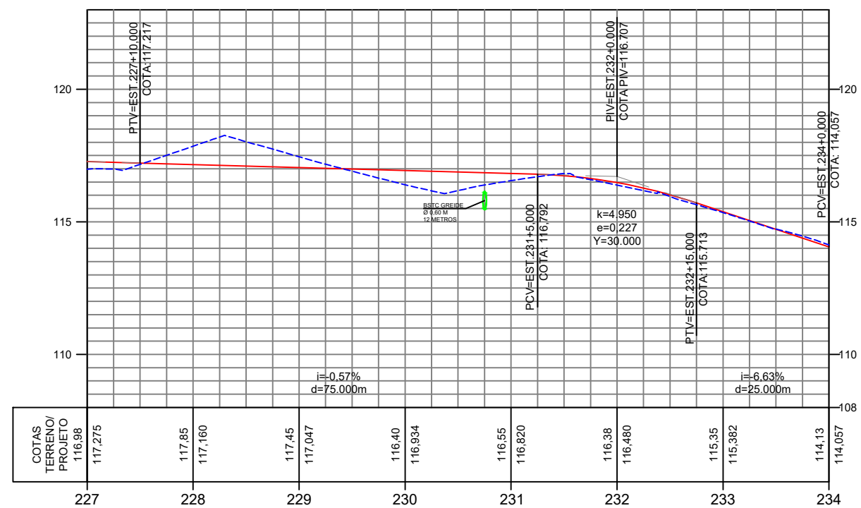
PERFIL LONGITUDINAL
