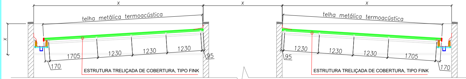
ESTRUTURA METÁLICA SEM ESCALA
