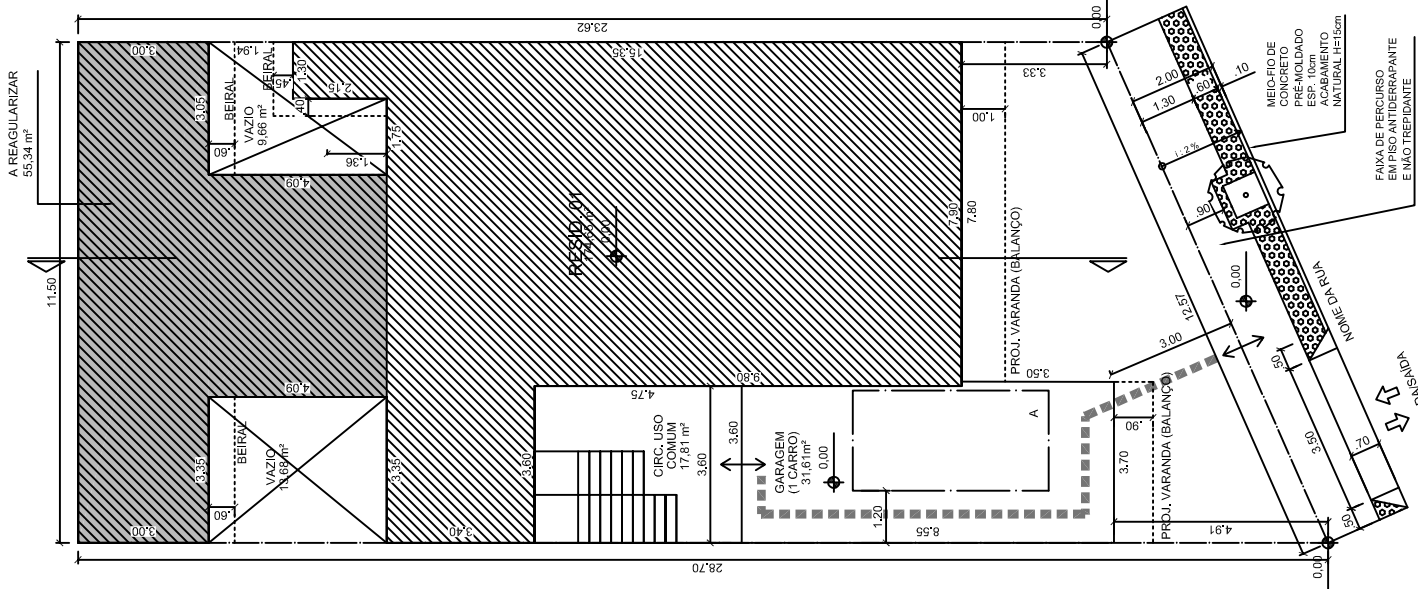
PLANTA 1º PAVIMENTO ESC.: 1/100
